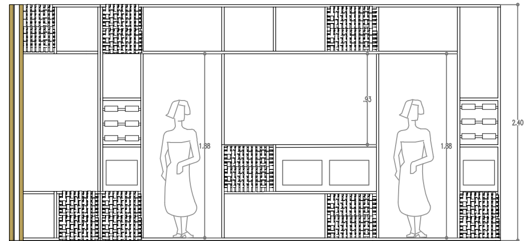
2 Sección longitudinal
