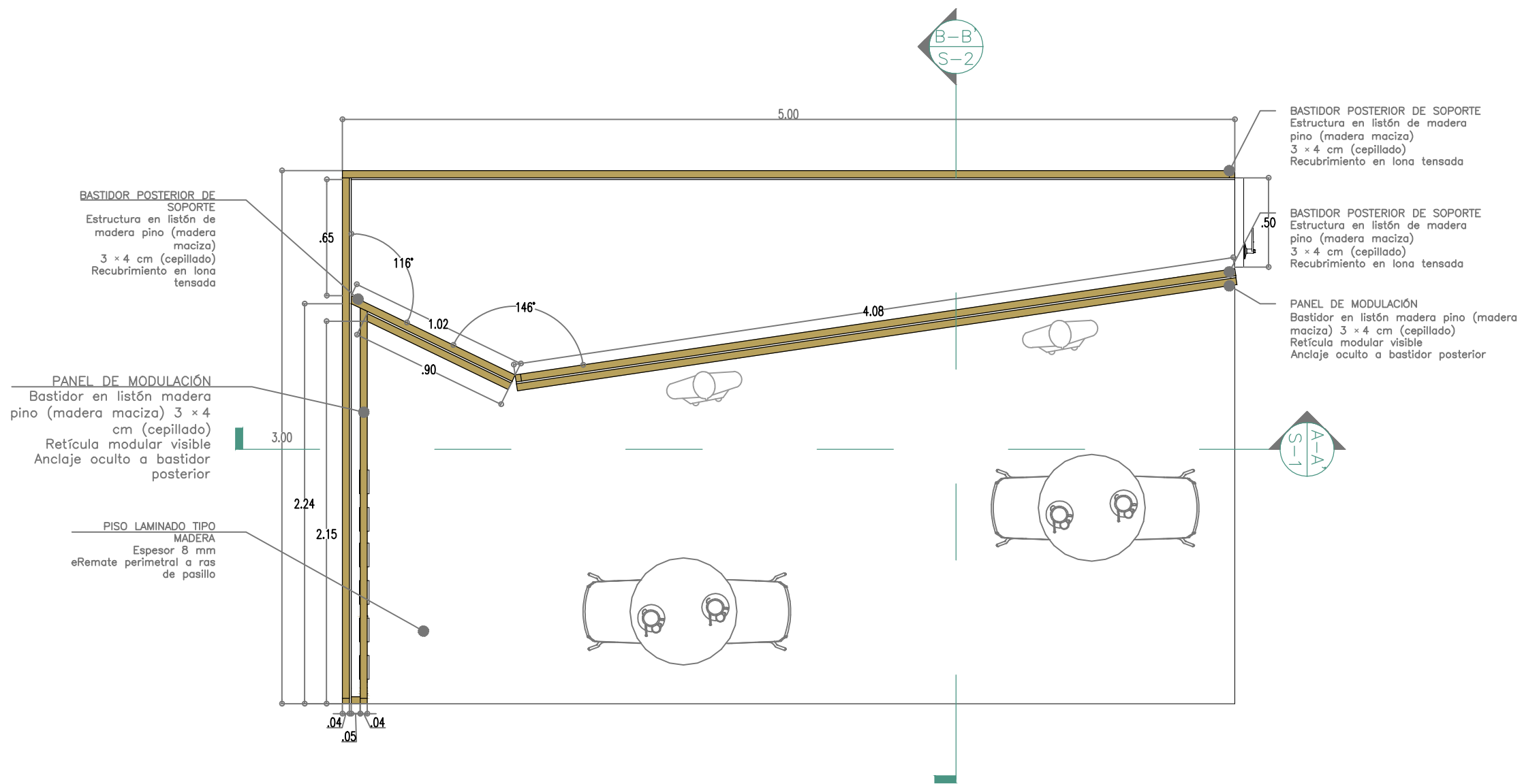
1 PLANTA
